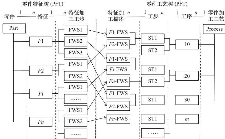
图1 特征加工工步与零件加工工艺中工步的对应关系
